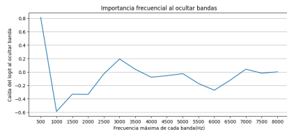
(a) Resultados de “logit” de la ocultación frecuencial en AASIST.
