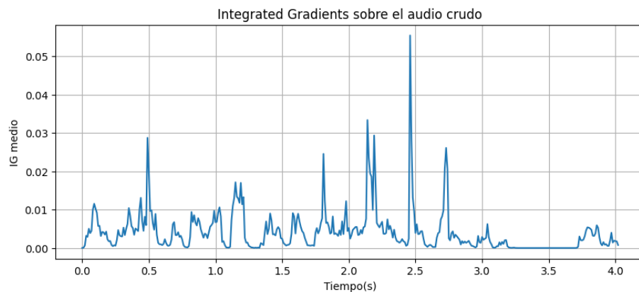
Figura 13: Importancia temporal según IG sobre audio.
